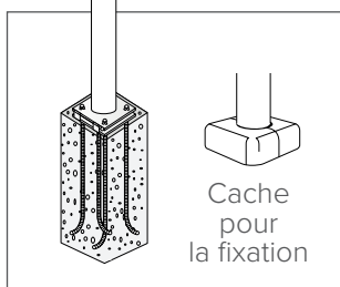
FSB - Fixation au sol basculante
