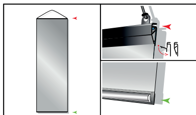
Système Klemmfix (latte en plastique renforcée d'une tige en acier) en haut, tige en fer dans l'ourlet du bas, corde en nylon transparente en haut.
