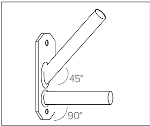
B36SR - Manchon mural droit, incliné
