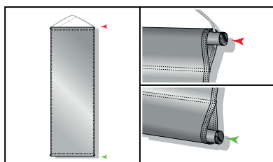
Tube en aluminium en haut et en bas avec bouchon de fermeture et corde dans le haut. Les tubes dépassent à gauche et à droite.
