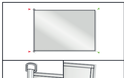
Sangle de renfort et anneaux-D, ourlets
